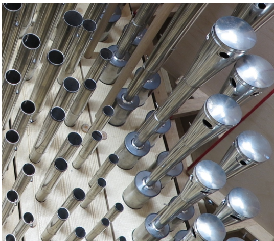
Pfeifenwerk
